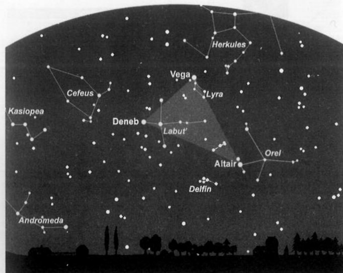
Mapka ukazuje situaci nad východním obzorem dne 15. července ve 22:00 hodin letního času. Na obrázku je vyznačen tzv. letní trojúhelník, v jehož vrcholech jsou nejjasnější hvězdy tří typicky letních souhvězdí - Lyry, Labutě a Orla.
